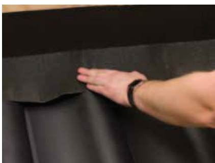
Aluflexen trykkes fast mod toppen af tagmaterialet.
