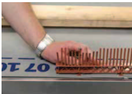
Fuglegitteret placeres på undertag og fodblik, så den hæver teglen ca. 20 mm over fodblikket.
