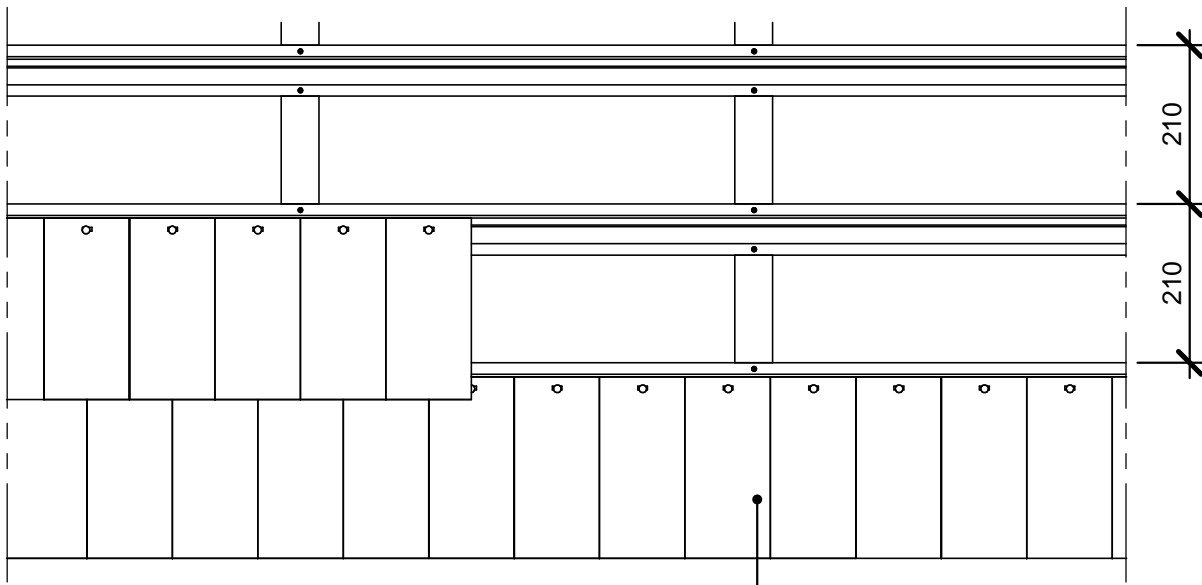
Elevation 1 : 10
