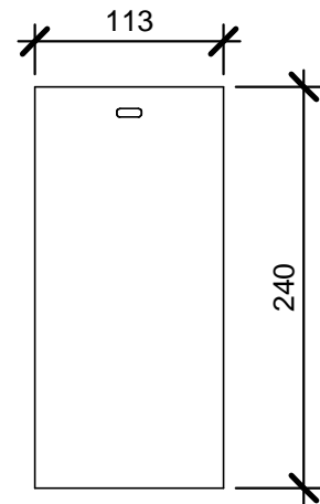
Clay Shingle 1 : 5
