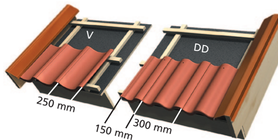
Figur 9. Opdel tagbredden i antal tagsten. Husk at den sidste sten ud mod ventre gavl dækker 330 mm for DD og 280 mm for V.
