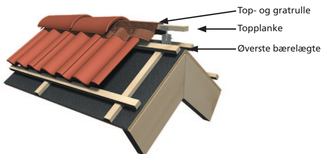
Figur 4. Afstanden fra topplankens centrum til øverste bærelægte skal være ca. 40 mm, se tabel 3. Afprøv, at rygningstenen overlapper øverste række tagsten på forsvarlig vis.
