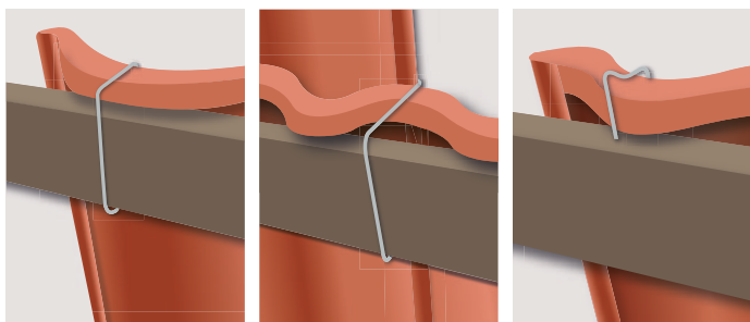
Figur 12a. Nakkeclips til fastgørelse af V og DD tagsten og specialsten.
