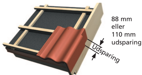
Figur 9. Opdel tagbredden i antal tagsten. Husk at den sidste sten ud mod ventre gavl dækker 330 mm for DD og 280 mm for V.
