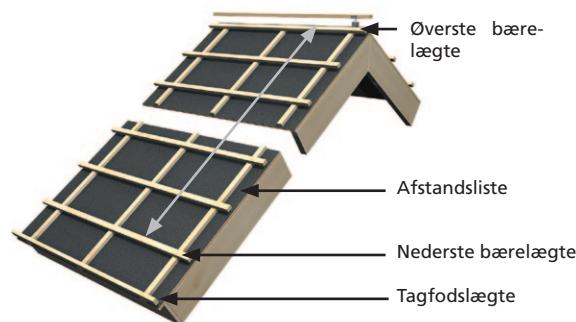
Figur 5. Udregn antallet af tagsten. Se også tabel 5.
