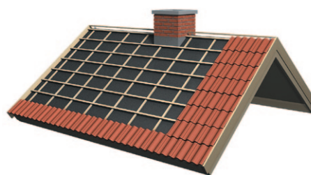
Figur 10. Læg nederste række fra højre mod venstre. Læg en hel række op i højre side til rygningen. Sørg for, at stenene ligger i vinkel. Når du har oplagt 2-3 rækker, kontrolleres om taget er i vinkel.
