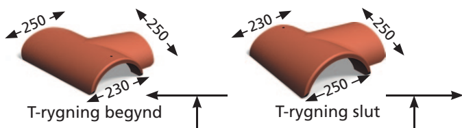
Figur 14. Anvendes hvor rygningerne mødes. Se tagretninger ovenfor.
