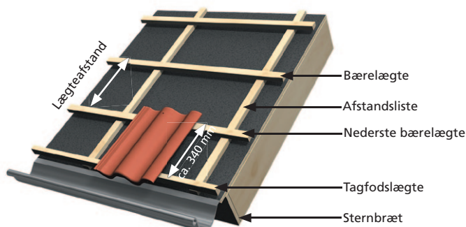
Figur 2. Lægteafstand måles fra overkant til overkant. Vær opmærksom på, at der fra tagfodslægtens nederste kant til nederste bærelægtes overkant ikke må være mere end 340 mm. Husk også på, at tagfodslægten skal være 20 mm højere end de øvrige bærelægter, da den nederste række tagsten ikke hviler på andre tagsten. Højdeforskellen kan udlignes ved brug af fuglegitter med ventilation.
