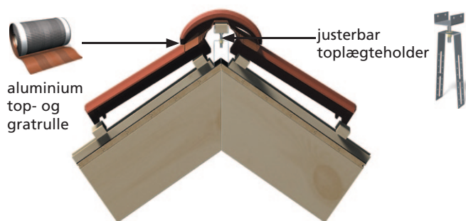
Figur 13. Anvendelse af KOMPROMENTs aluminium top- og gratrulle. Let at montere, skal blot rulles ud over toplægten, og lægges ned over de øverste rækker tagsten, hvorefter beskyttelsespapiret fjernes og rullen presses ned i tagstenens bølger.
